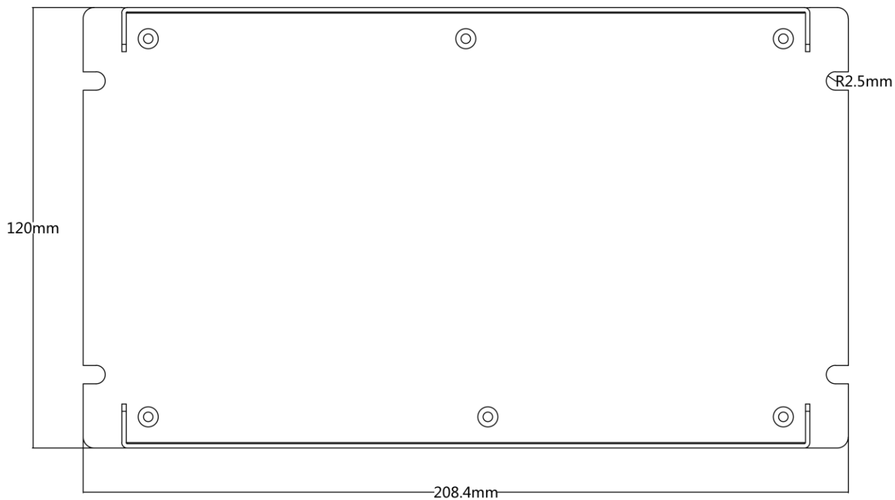
HK-6D-U402 尺寸图
