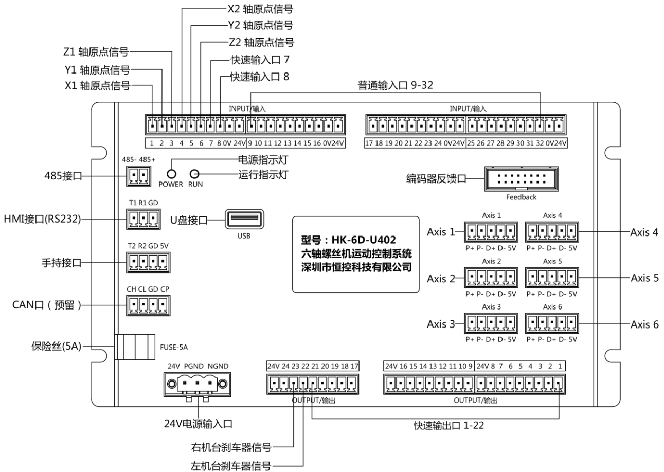
HK-6D-U402 接口示意图
