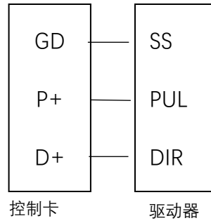
共阴极接线图：
