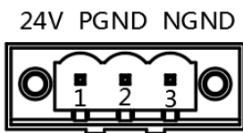
电源输入口
